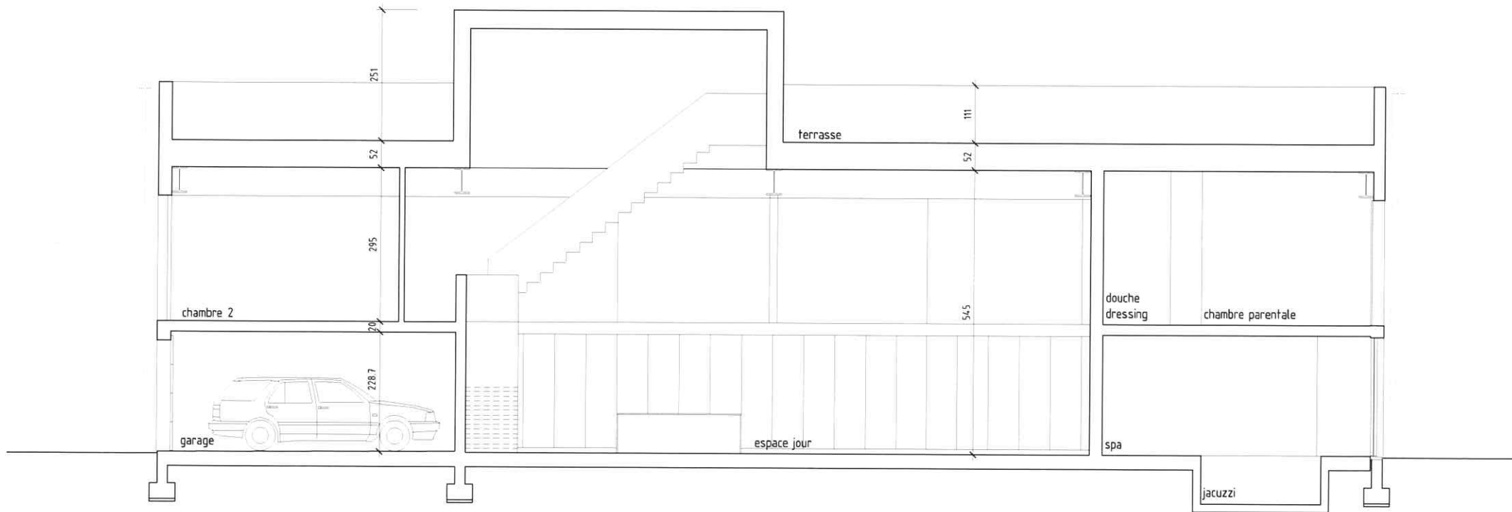
coupe A-A
